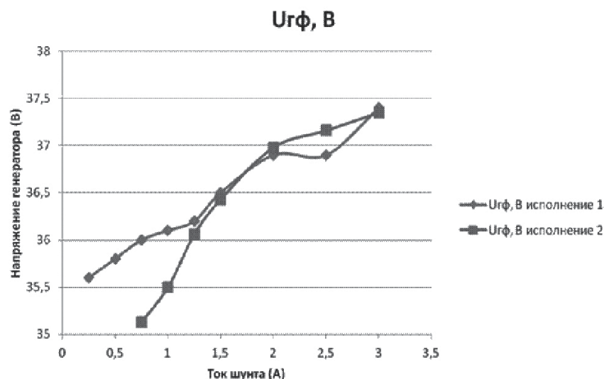
Рисунок 2 – Характеристики холостого хода модели магнитоэлектрического генератора
