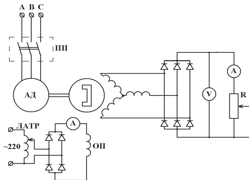
Рисунок 1 – Схема модели трехфазного магнитоэлектрического генератора
